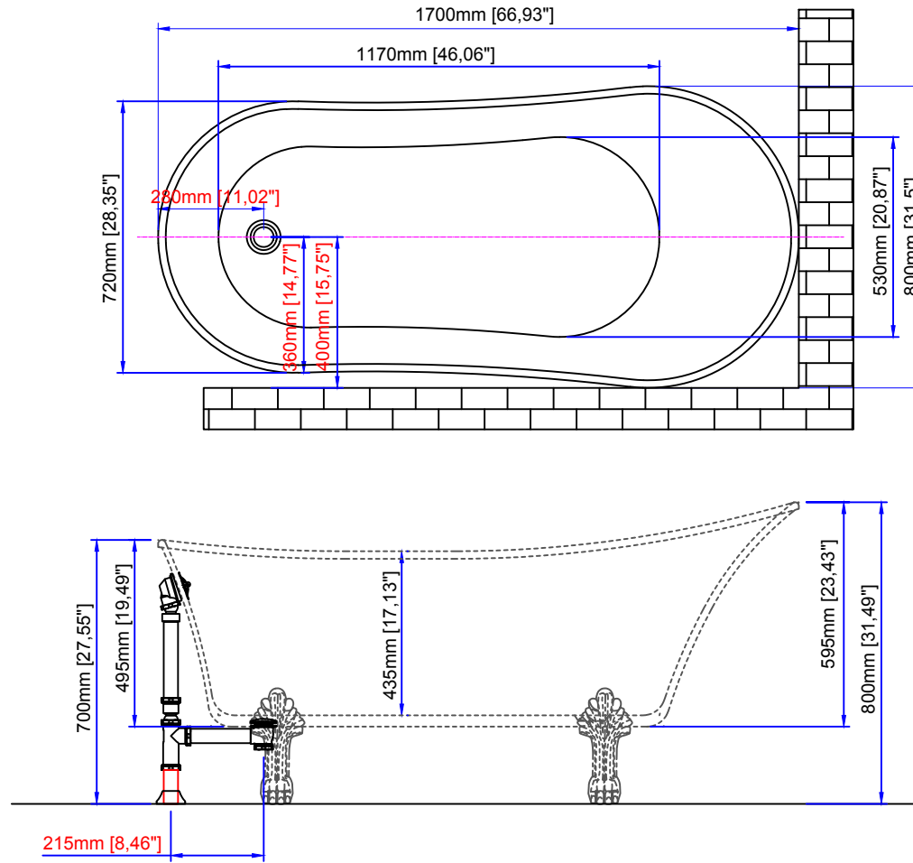
N-340-67CFWH-FM
